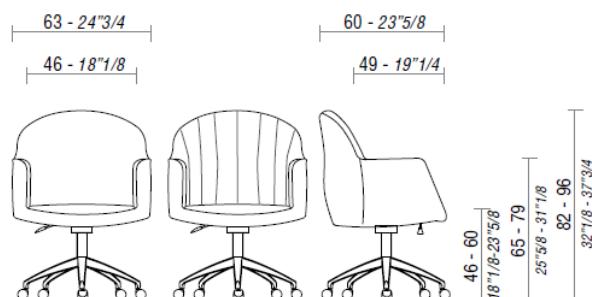
TULIP, POLTRONA CON SCHIENALE BASSO TULIP, CHAIR WITH LOW BACKREST
