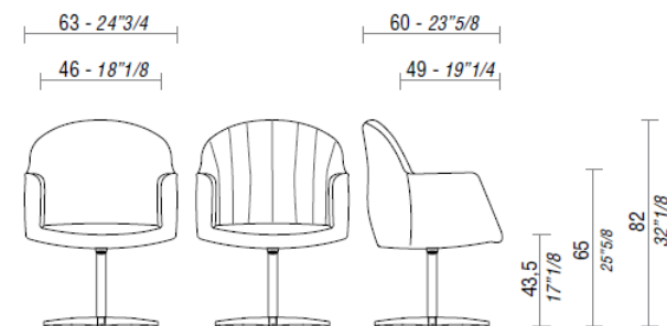
TULIP, POLTRONA BASE A CROCE CON SCHIENALE BASSO TULIP, CHAIR WITH CROSS-SHAPED BASE AND LOW BACKREST
